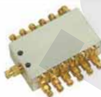
CV型單一循環分配器 CV Progressive Feeders
